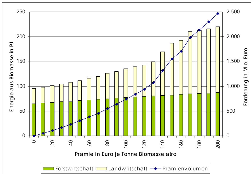
Abbildung 1: Ergebnisse der Simulationsberechnungen: zusätzliche organische Trockenmasse aus der Land- und Forstwirtschaft in Abhängigkeit vom Umfang der Förderung (in € je Tonne Trockenmasse für die energetische Verwertung)
